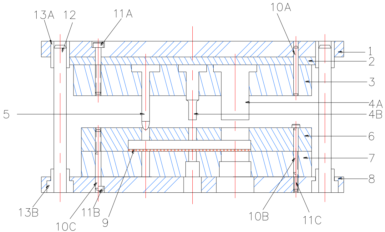
圖、沖壓模具之薄殼大量生產件結構示意圖
